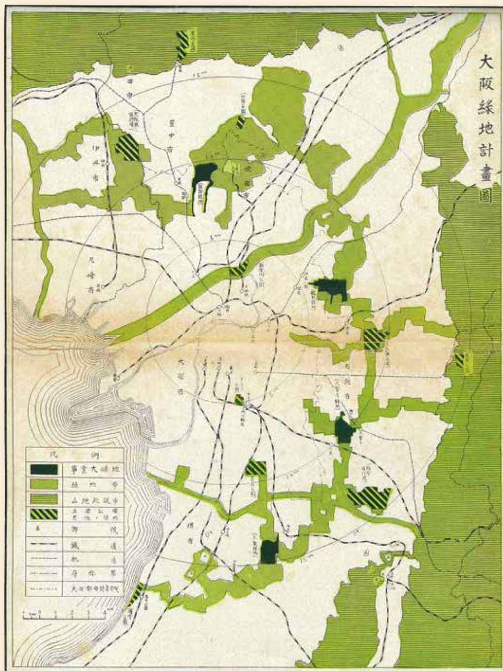
大阪緑地計画図(昭和16年告示)
